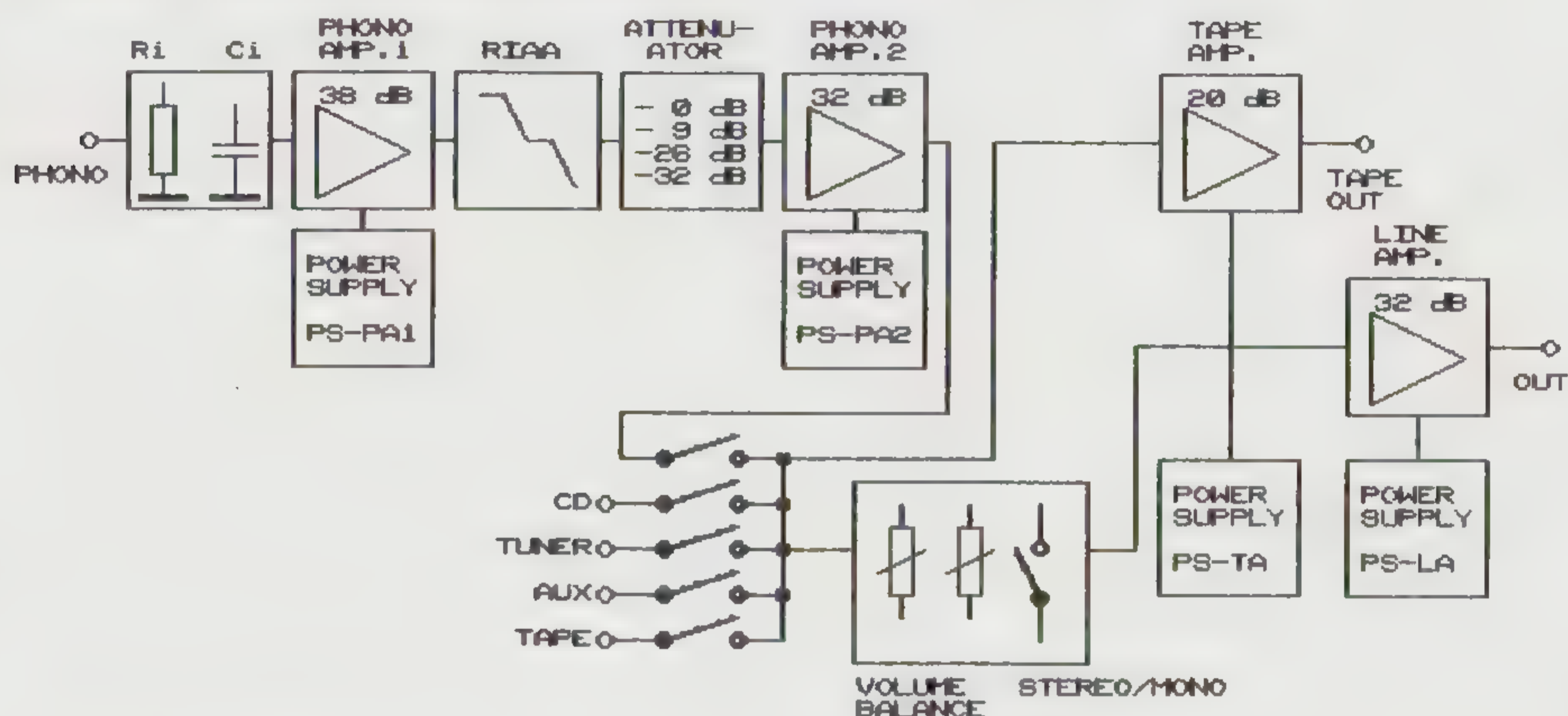
Figuur 9 Blokschema
